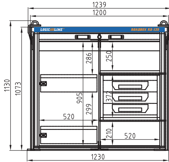
Beifahrerseite
