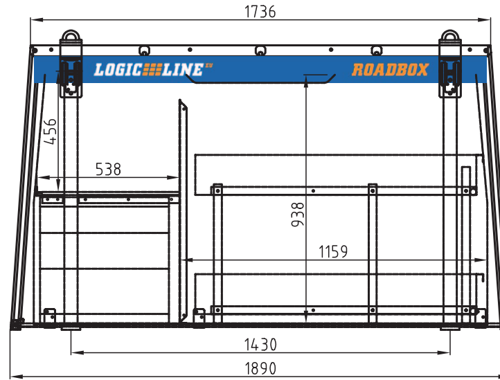
Ansicht Heck
