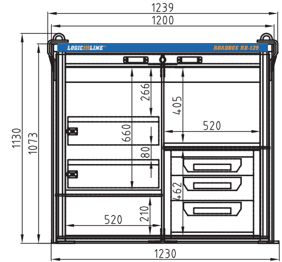
Fahrerseite
