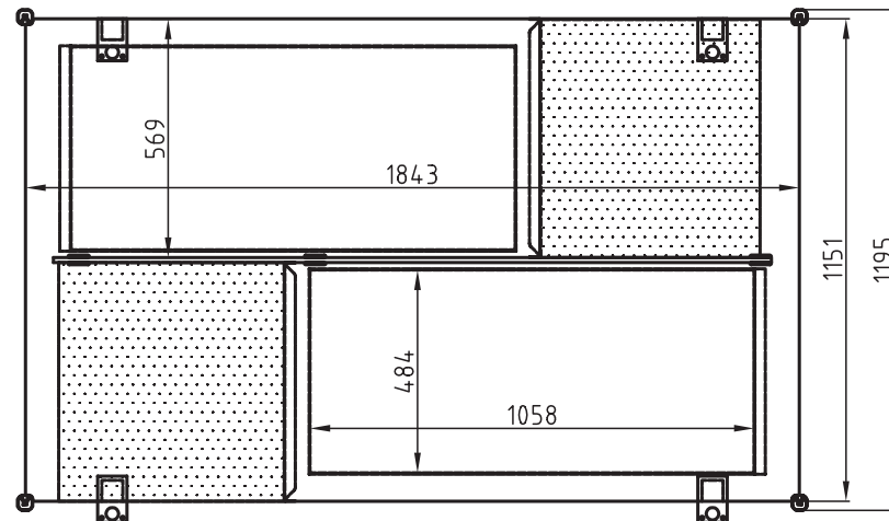
Draufsicht
