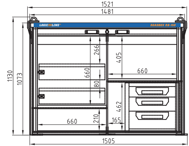
Fahrerseite
